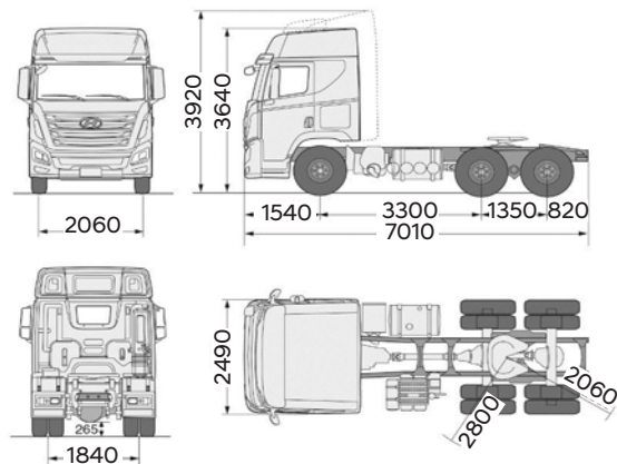
Largo / Ancho / Altura / Distancia entre ejes (mm)
